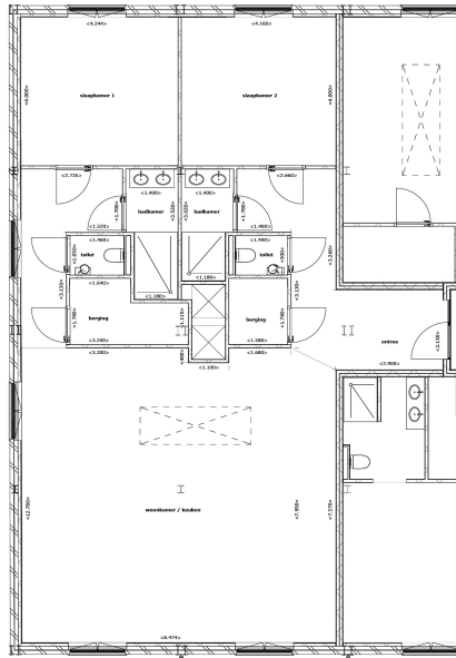
Plattegrond verdieping 03 1:50
